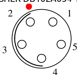
Rys. 2.1. Gniazdo mikrofonowe - widok z zewnątrz.
