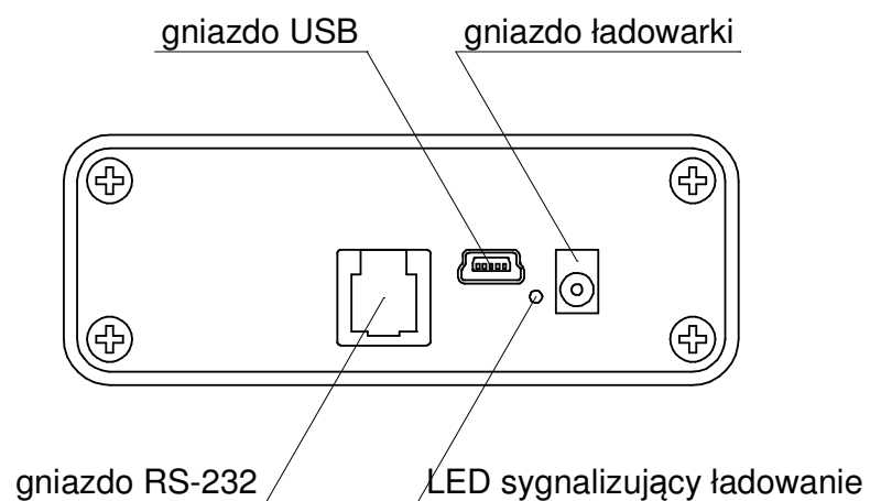
Rys. 1.2. Miernik poziomu dźwięku DLM-101 - widok panelu dolnego.
