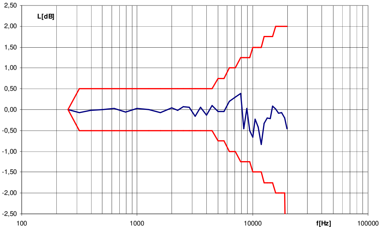
Rys. 1.5. Typowa charakterystyka skuteczności mikrofonu WK-21 w polu swobodnym.
