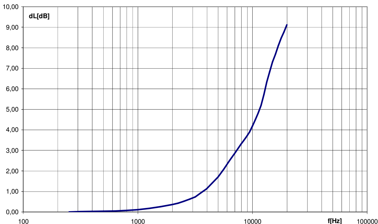
Rys. 1.4. Poprawka pola swobodnego dla mikrofonu WK-21 i kierunku 0°.
