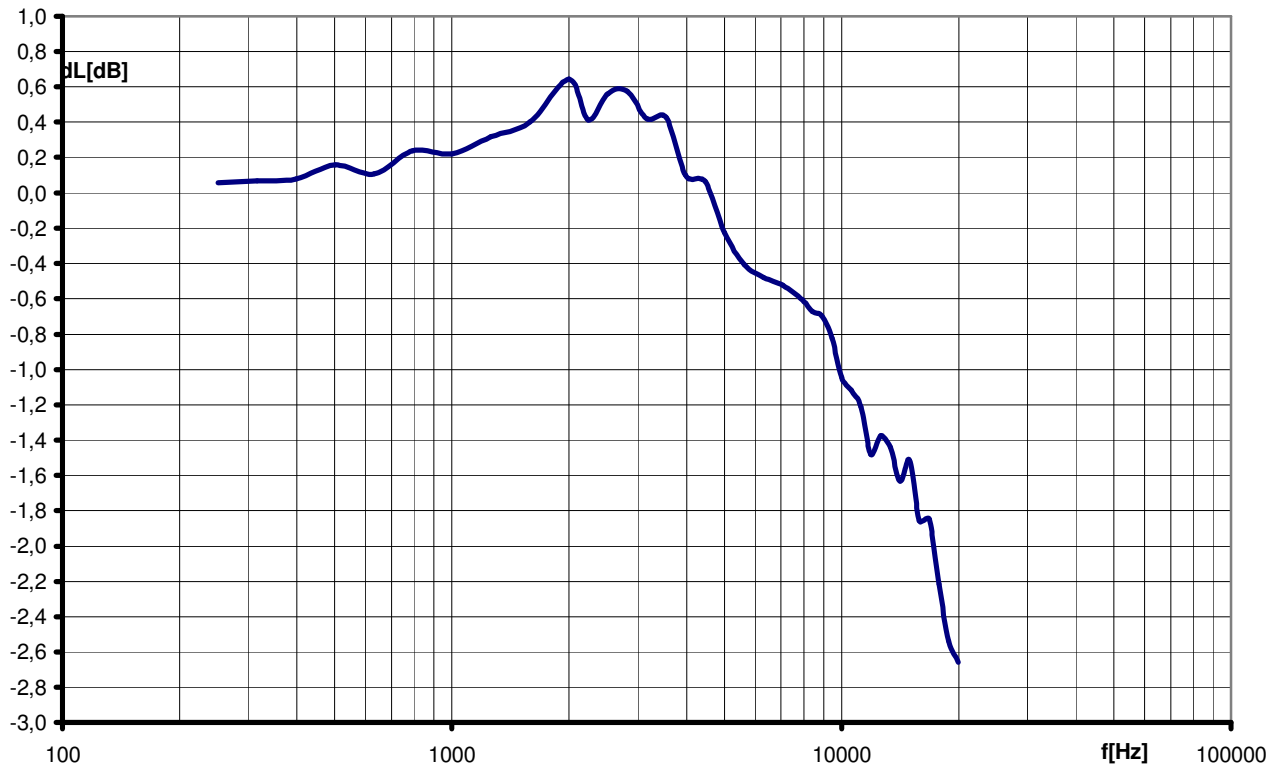
Rys. 1.6. Wpływ osłony przeciwwietrznej OP60/2.
