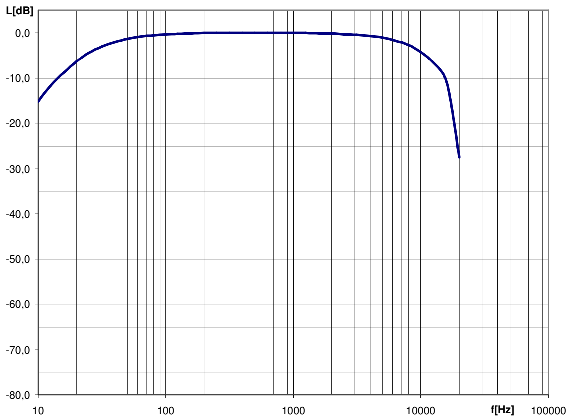
Rys. A.2. Charakterystyka filtru C, zgodnego z PN-EN 61672-1:2014, klasa 1.
