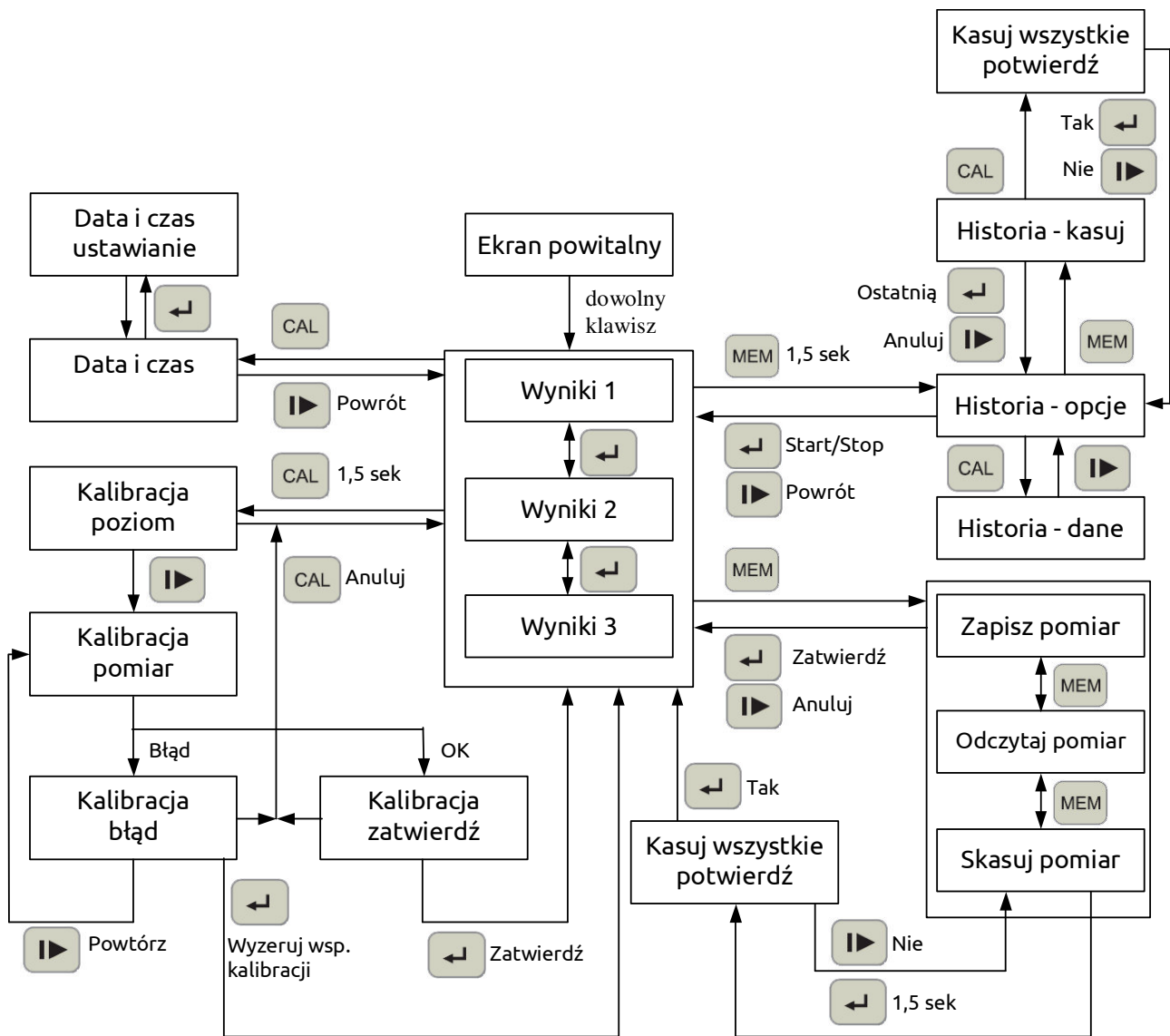
Rys. 3.1. Schemat przejść między ekranami menu.
