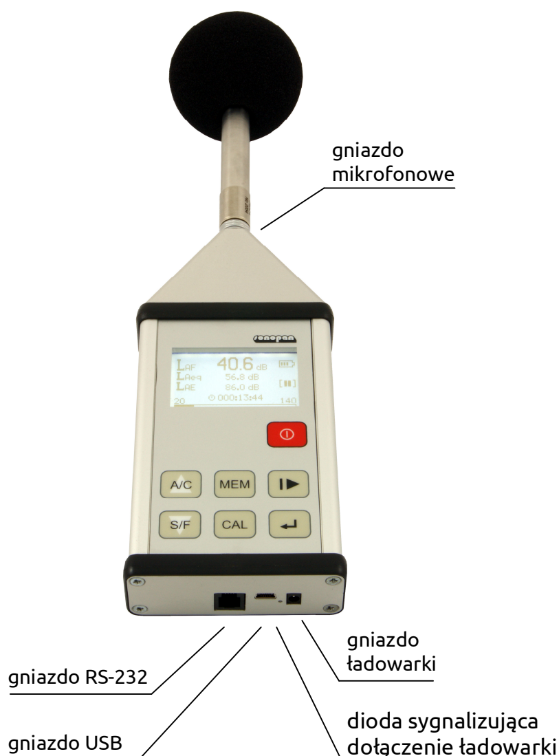
Rys. 1.1. Miernik poziomu dźwięku DLM-101 - widok ogólny.
