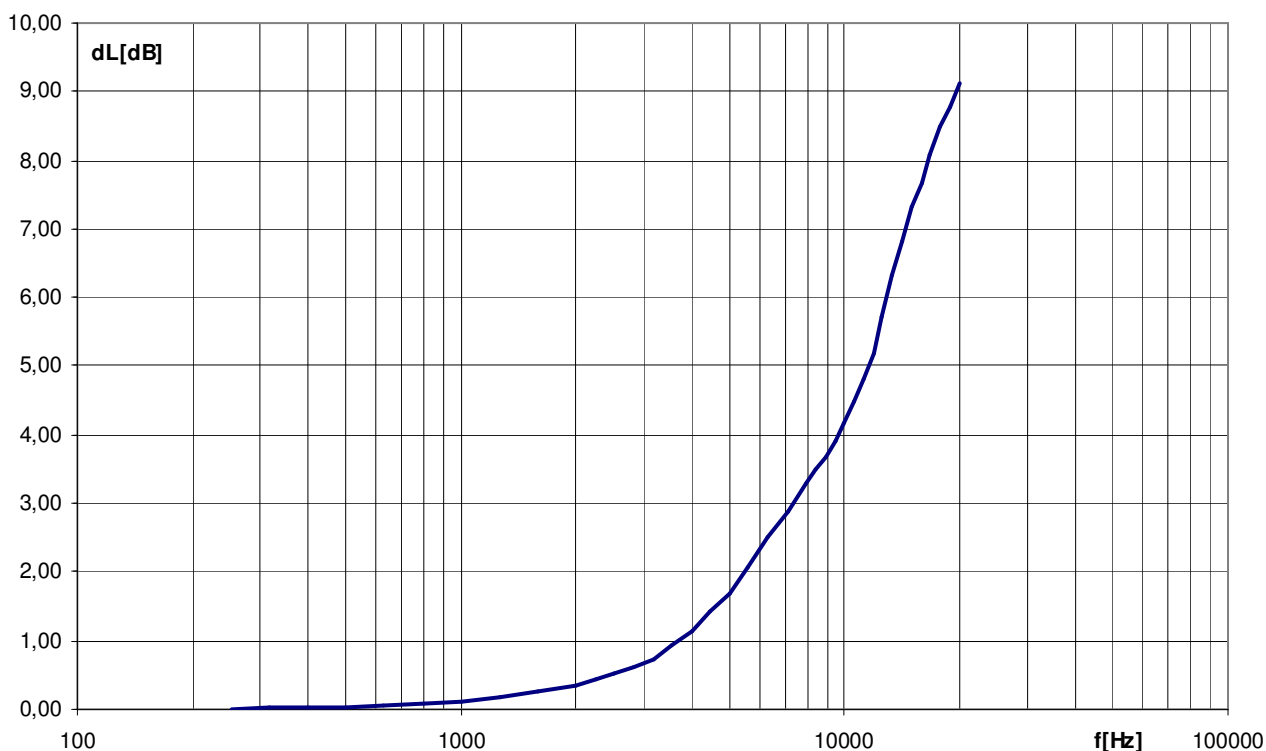
Rys. 1.3. Poprawka pola swobodnego dla mikrofonu WK-21 i kierunku 0°.
