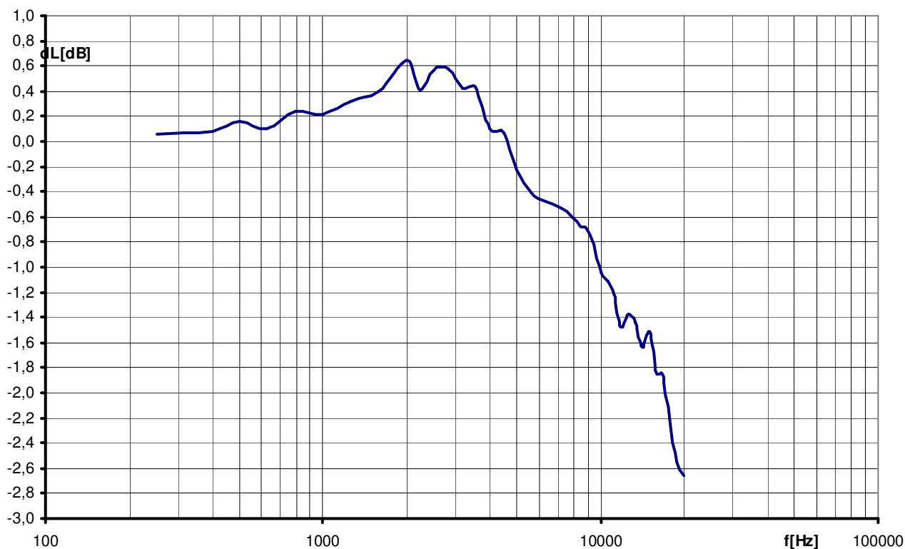
Rys. 1.5. Wpływ osłony przeciwwietrznej OP60/2.
