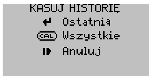
Rys. 3.15. Historia – kasowanie.
