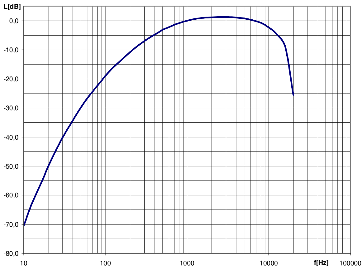
Rys. A.1. Charakterystyka filtru A, zgodnego z PN-EN 61672-1:2014, klasa 1.
