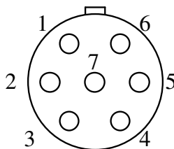
Rys. 2.1. Gniazdo mikrofonowe - widok z zewnątrz.
