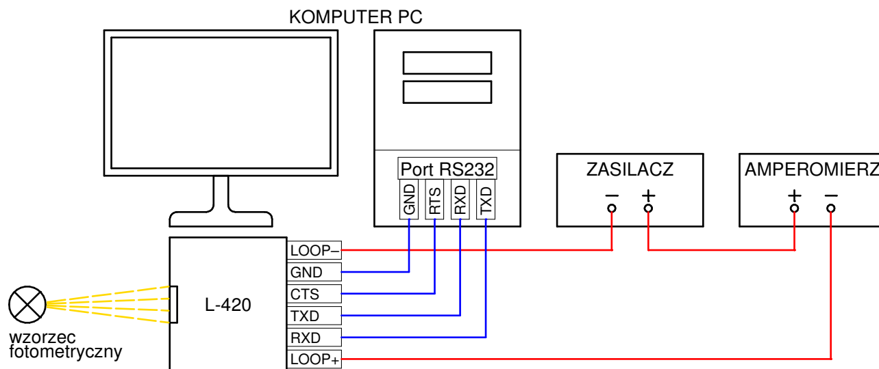
Rys. 2. Schemat układu kalibracji.
